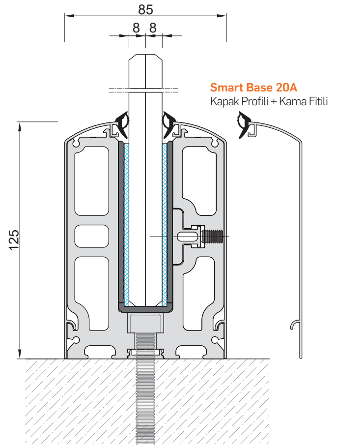
SMART BASE 85-125A CAMLI KORKULUK SİSTEMİ 8 mm + PVB + 8 mm
