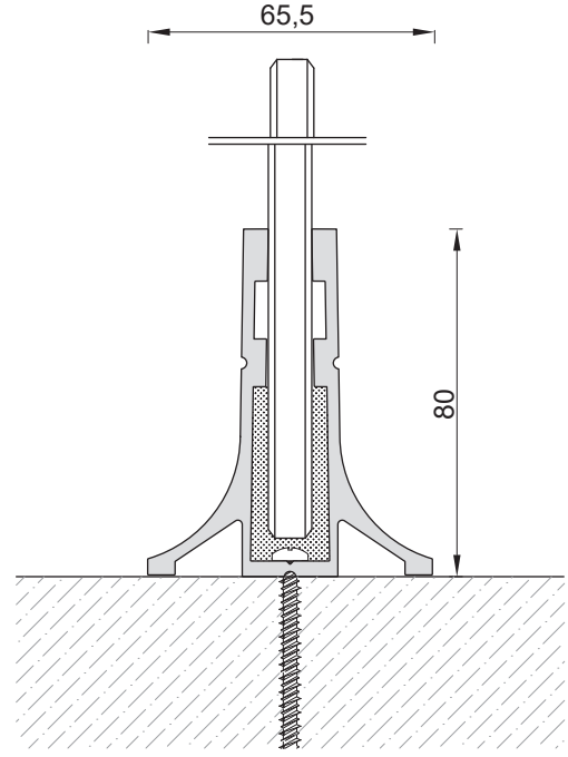
SLIM BASE CAMLI KORKULUK SİSTEMİ 10 mm
