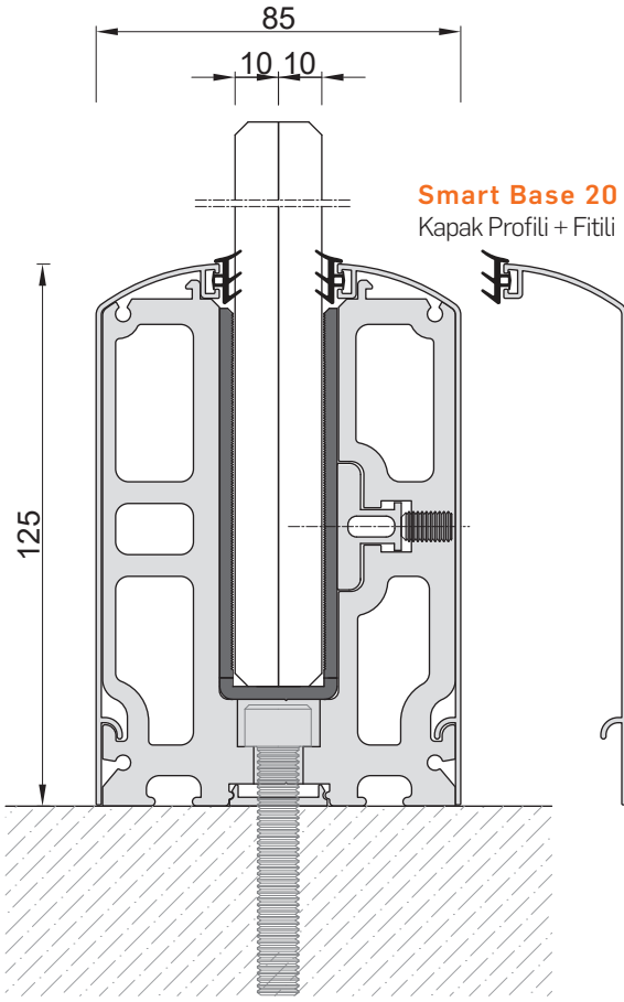
SMART BASE 85-125 CAMLI KORKULUK SİSTEMİ 10 mm + PVB + 10 mm
