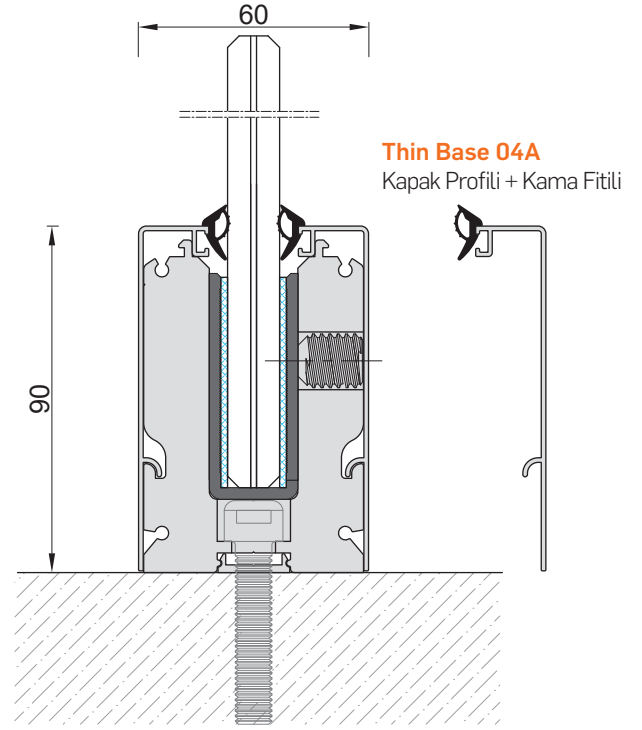
THIN BASE 90A CAMLI KORKULUK SİSTEMİ 6 mm + PVB + 6 mm
