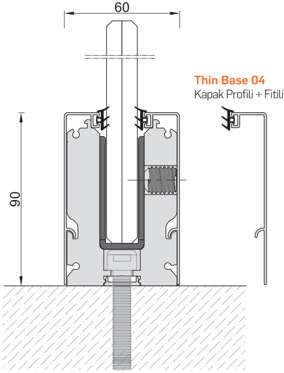
THIN BASE 90 CAMLI KORKULUK SİSTEMİ 8 mm + PVB + 8 mm
