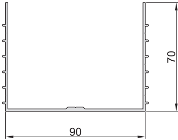
Smart Base 30 Kanal Profili
