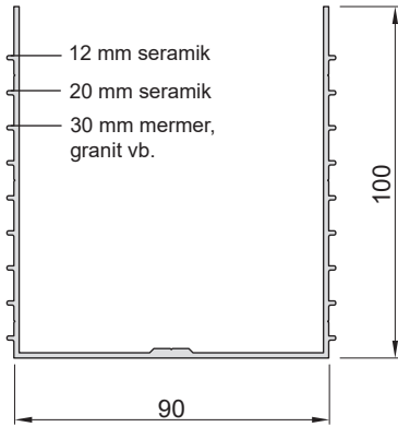
Smart Base 28 Kanal Profili
