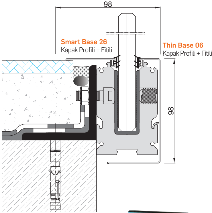
THIN BASE 90B CAMLI KORKULUK SİSTEMİ 8 mm + PVB + 8 mm
