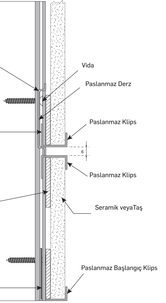
DÜŞEY KESİT
