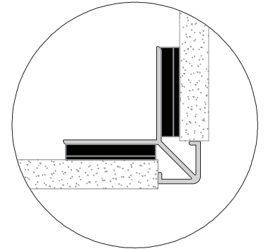
A Detayı
