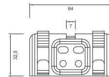
Tekli Klips
